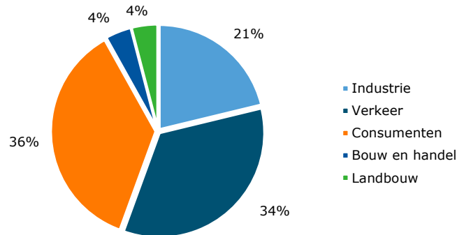
Figuur 2 Aandeel sectoren in emissie van fijnstof PM2,5 (jaar 2020)
