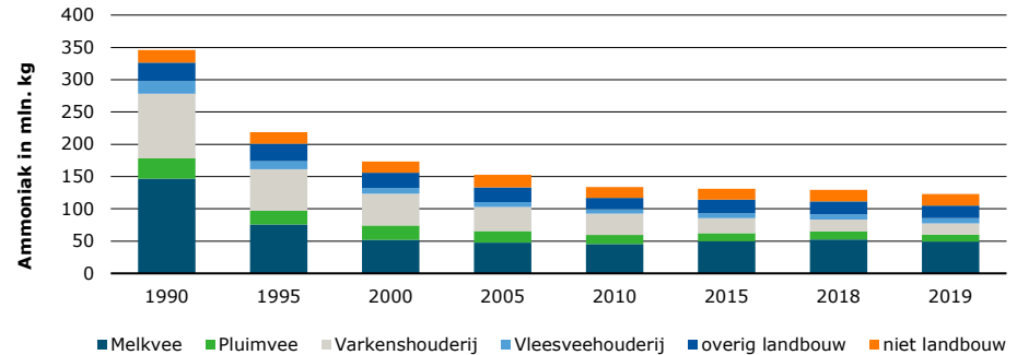
Figuur 1 Ontwikkeling ammoniakemissie per sector
